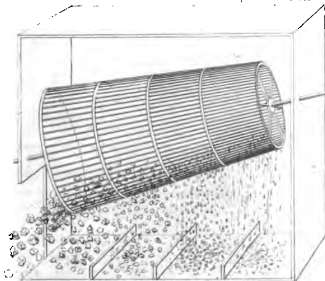
Cylinder for washing the Cascalhão. p. 333.
